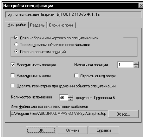
Рис. 16.1. Общие настройки спецификации
