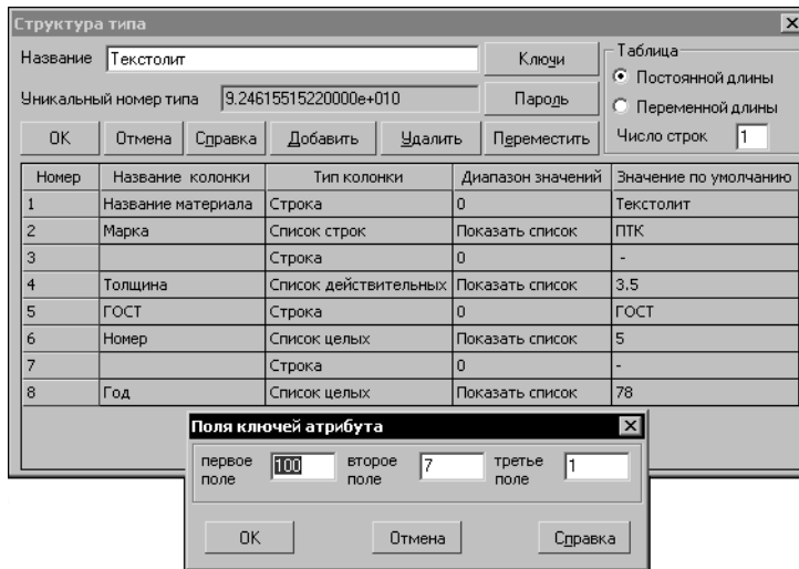
Рис. 20.7. Новый тип атрибута (шаблон заполнения обозначения текстолита)
